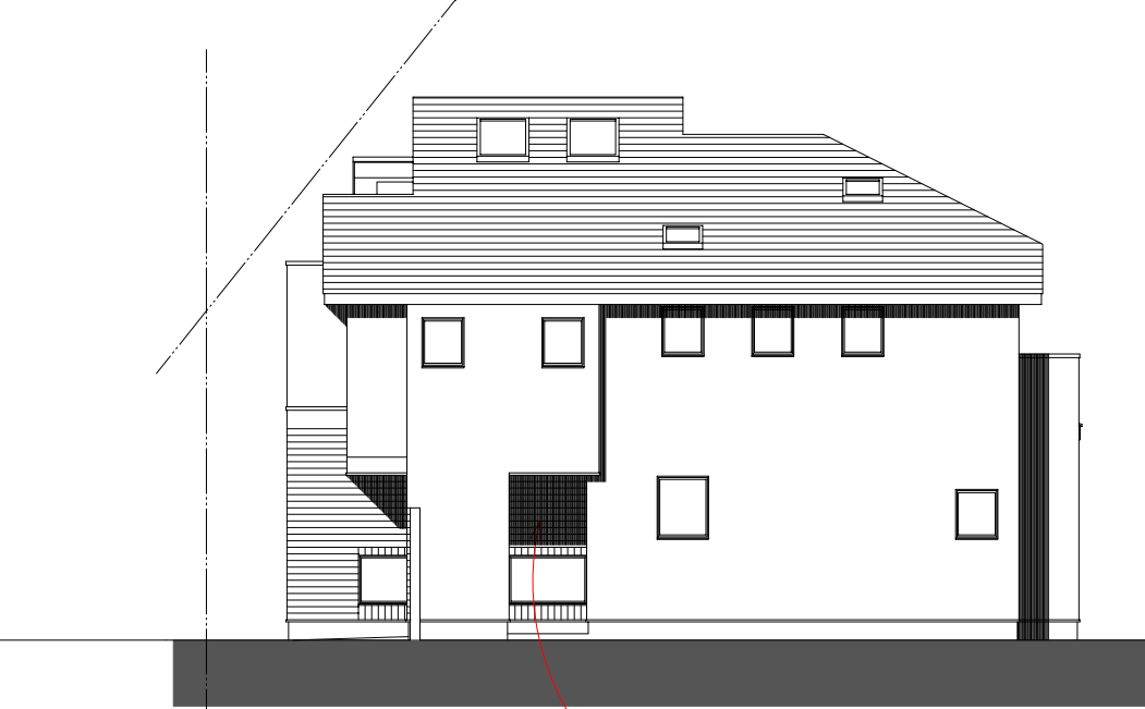
期 北側立面図 S = 1/100
